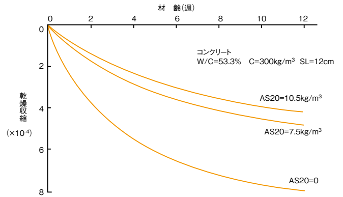
● テトラガードを用いたコンクリートの乾燥収縮
