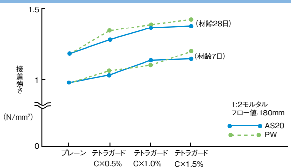
● テトラガードを用いたモルタルの接着強さ
