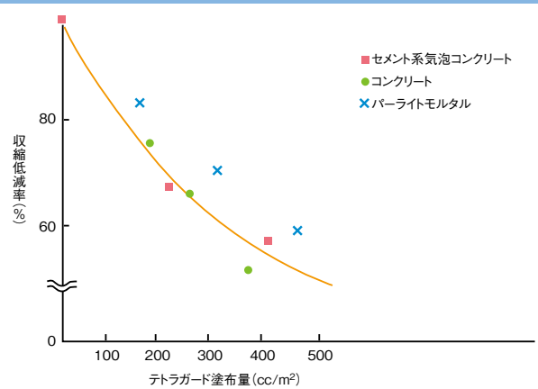
● テトラガード塗布量と乾燥収縮低減率の関係
