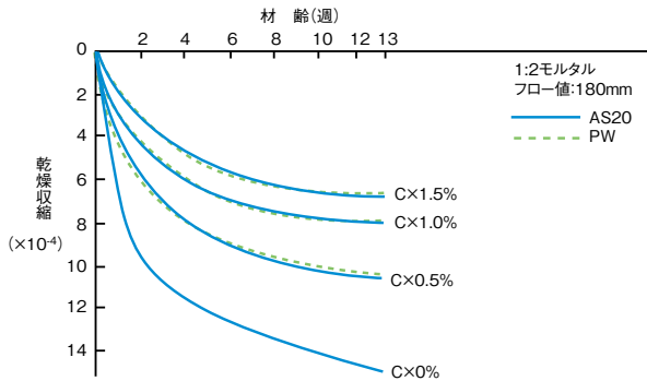
● テトラガードを用いたモルタルの乾燥収縮
