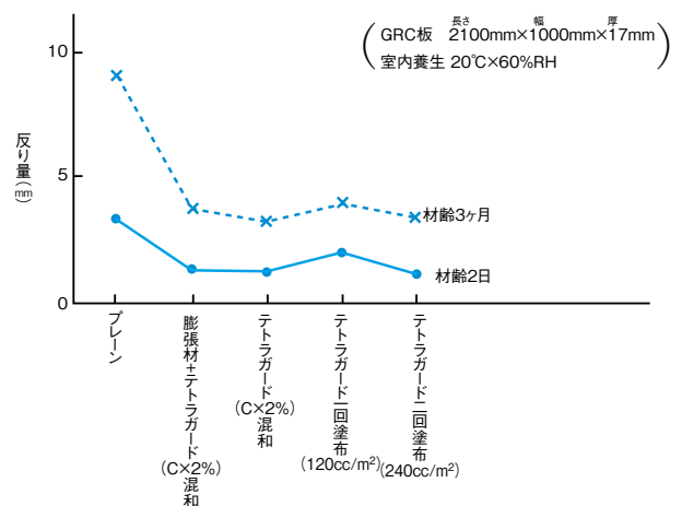
● テトラガードを用いたGRC板の反り量
